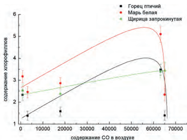
Рис. 4. Зависимость показателя суммарного содержания хлорофиллов (мг/г сухой массы) растений урбофитоценозов от концентрации CO 2 в воздухе (мг/м 3 ).
